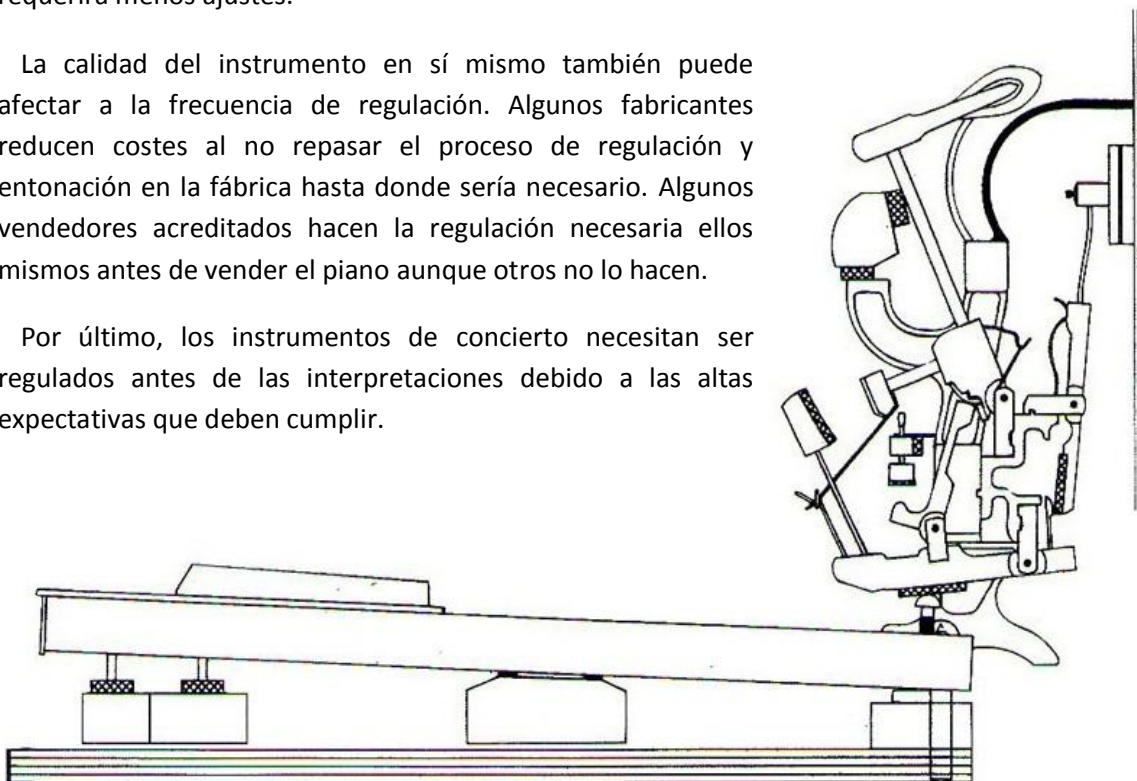
Acción de un piano vertical. Cada nota tiene más de 25 puntos de ajuste.
