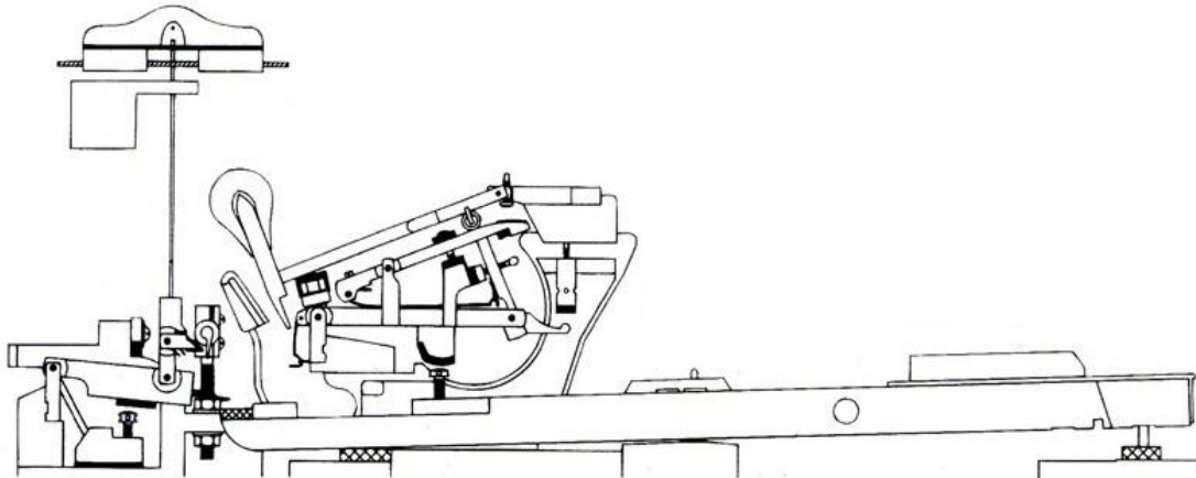
Acción de un piano de cola. Cada nota tiene más de 35 puntos de ajuste.
